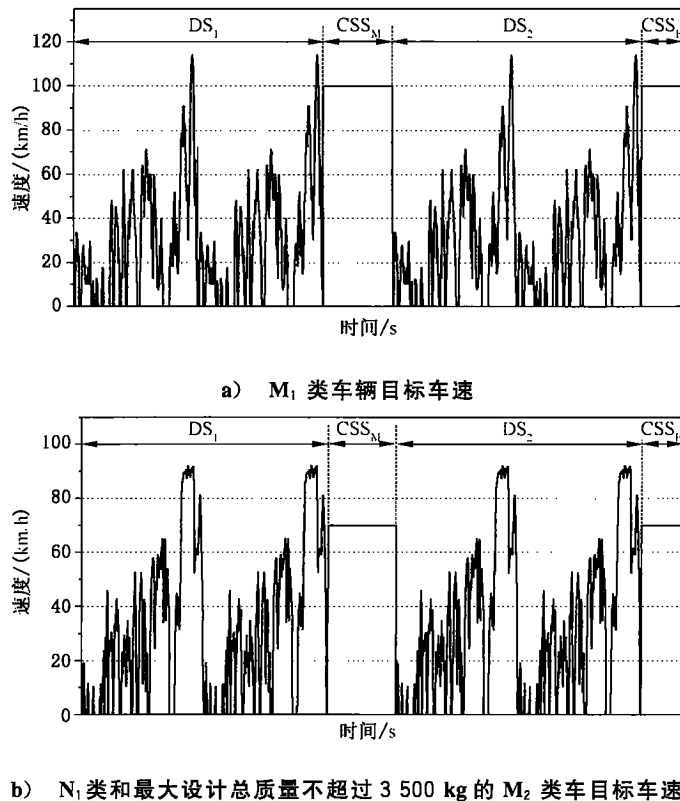
图 1 缩短法速度片段构成
